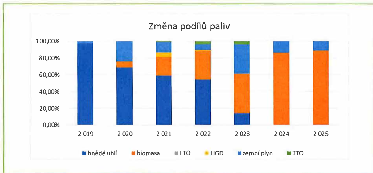
Obr. 4: Změna využití paliv
