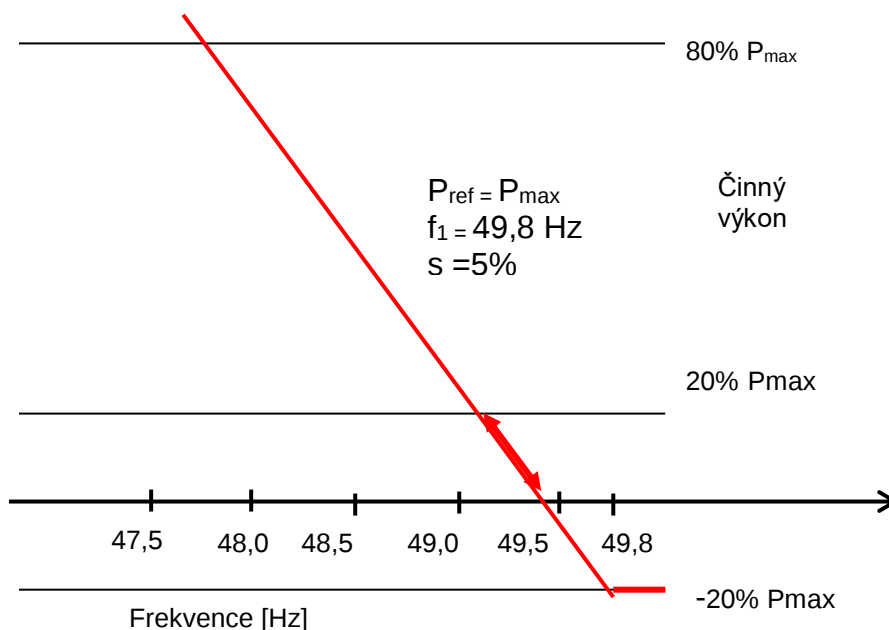
Obr.7 Frekvenční odezva činného výkonu na podfrekvenci u akumulčního zařízení.
