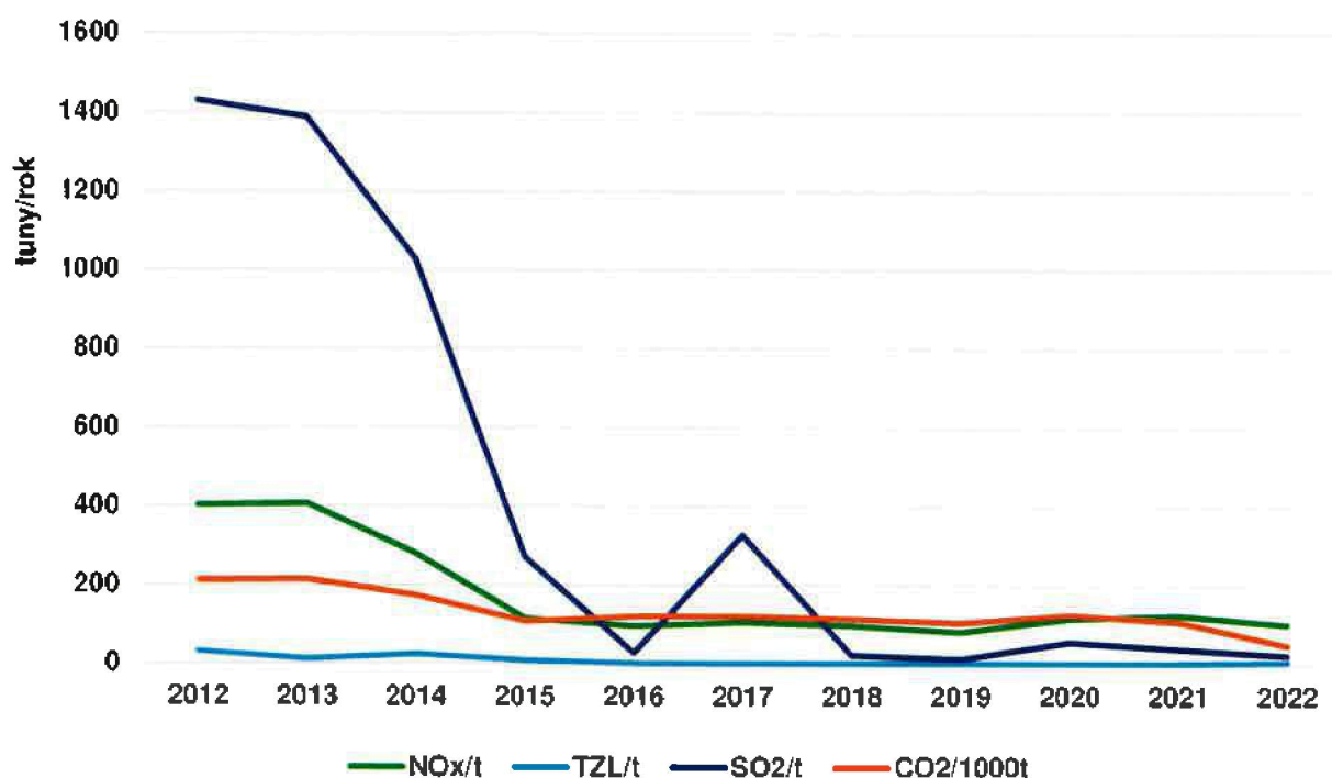
Graf 3: Přehled produkce emisí v C-Energy Planá
